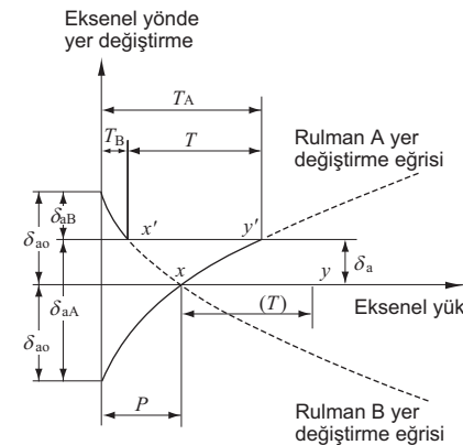
Şekil 11-1 Pozisyon önyüklemede önyükleme şeması
