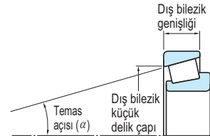
ISO altı birim spesifikasyonları
