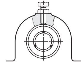
Şekil 1 Boşluk ayarı
