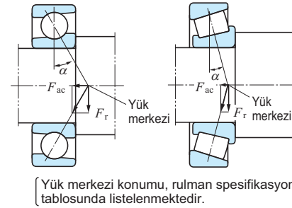
Şekil 5-11 Eksenel bileşen kuvveti
