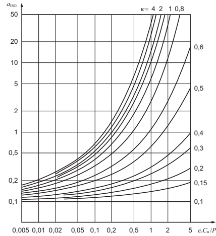
Şekil 5-3 Ömür düzenleme faktörü a_{ISC} (Radyal makaralı rulmanlar)
