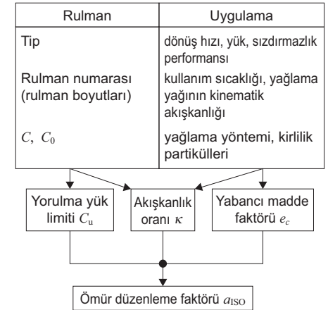
Şekil 5-1 Sistem yaklaşımı
