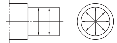
Şekil 15-1 Mil çapındaki ölçüm noktaları
