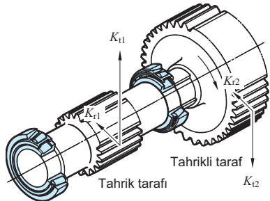
Şekil 5-7 Düz dişliler üzerinde yük
