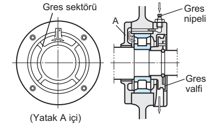
Şekil 12-1 Gres besleme yöntemi örneği (gres sektörü kullanma)
