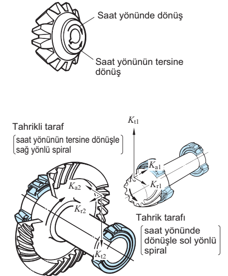
Şekil 5-10 Spiral konik dişliler üzerindeki yük
