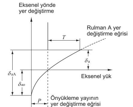
Şekil 11-2 Faktör basıncıyla önyüklemede önyükleme şeması
